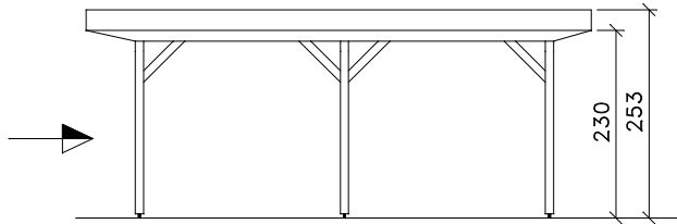
Seitenansicht
