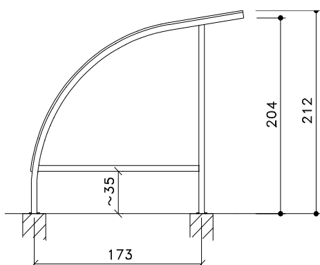
Vue latérale
