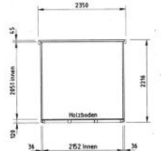
Querschnitt
